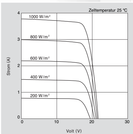
Strom-Spannungs-Kennlinie des Moduls KC60 bei verschiedener Einstrahlung.
