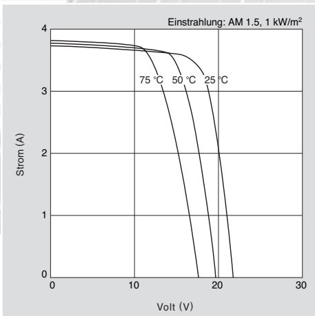
Strom-Spannungs-Kennlinie des Moduls KC60 bei verschiedenen Zelltemperaturen.
