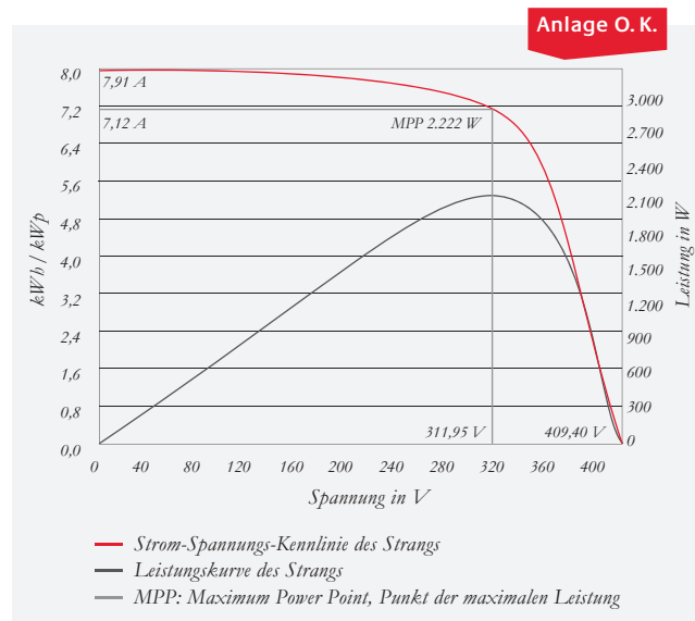
Kennlinienmessung
