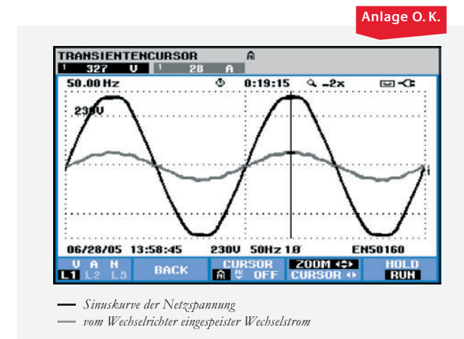
Wechselrichterüberprüfung
