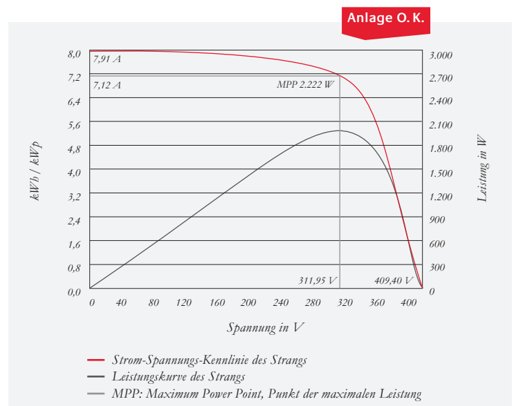
Kennlinienmessung
