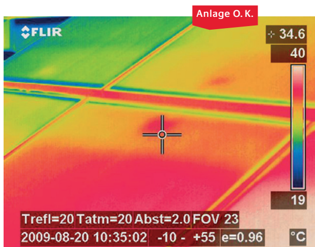
Infrarotmessung
